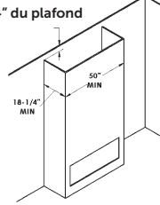
Charpente jusqu'au plafond avec aération à l'avant ou sur les côtés
