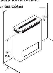
Enchâssure minimale avec aération à l'avant ou sur les côtés
