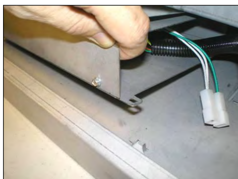
2. Soulevez la boîte UHS et sortez-la de l'appareil.
