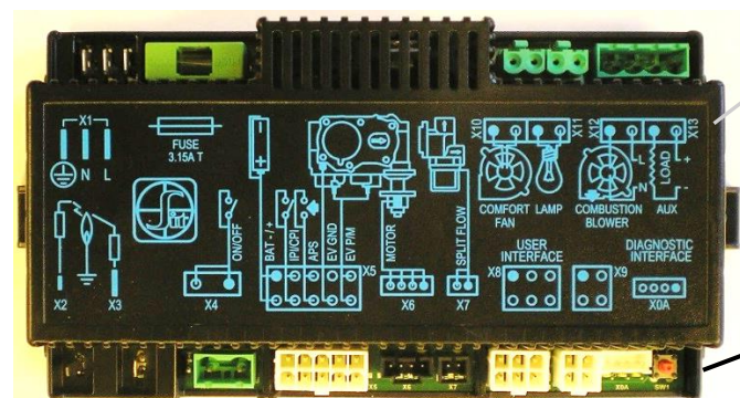
IFC Module
