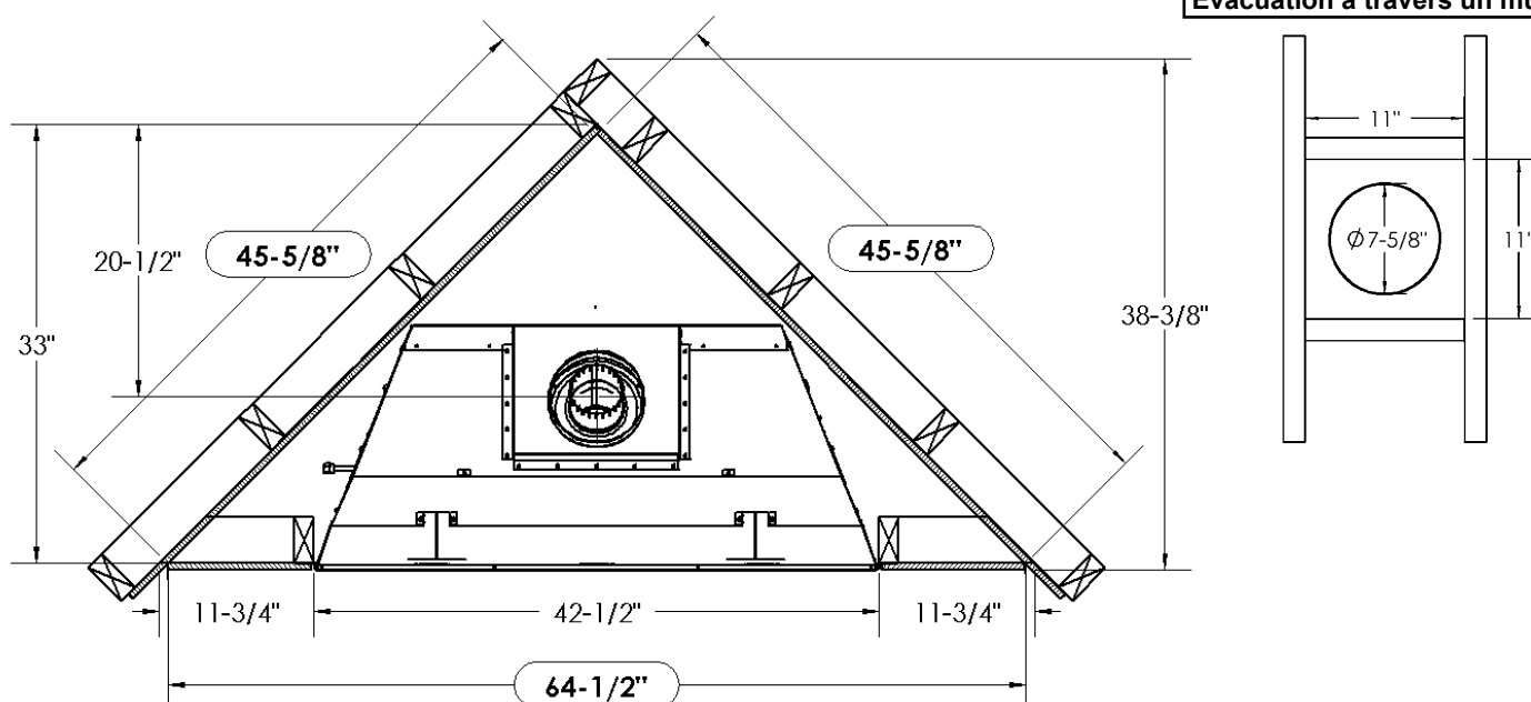
Fig. 1 Charpente l'évacuation horizontale (Voir la section Évacuation à travers un mur)
