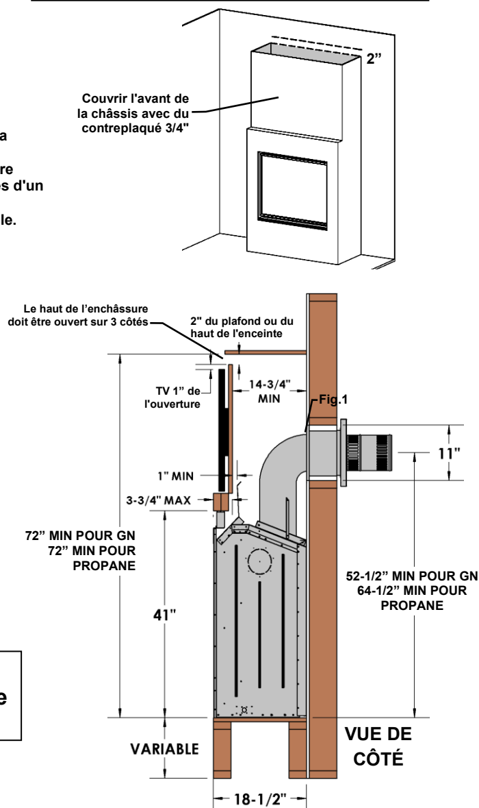
Fig. 1 Charpente l'évacuation horizontale (Voir la section Évacuation à travers un mur)
