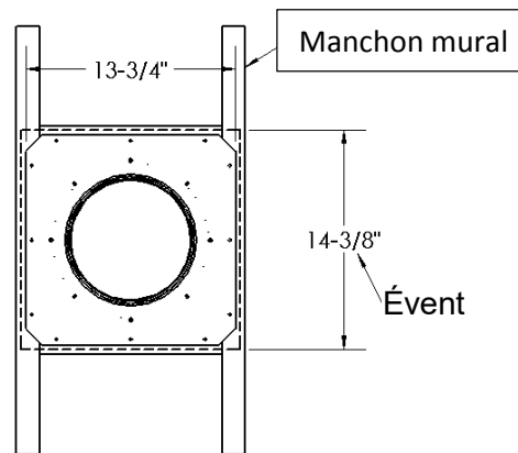
Nouveau manchon mural Nouvel évent
