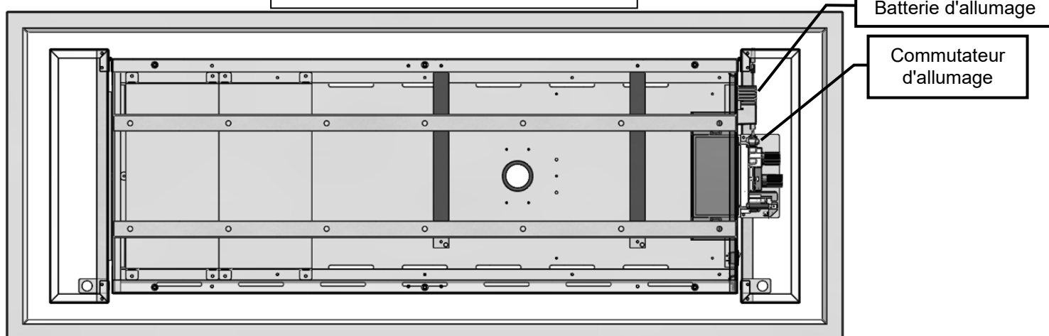
OLTG/ OLTB – Vue de dessus
