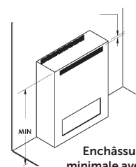
Charpente jusqu'au plafond avec ouverture avant
