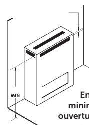
Enchâssure minimale avec ouvertures avant et arrière
