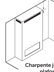
Enchâssure ouverte avec distance minimale au plafond
