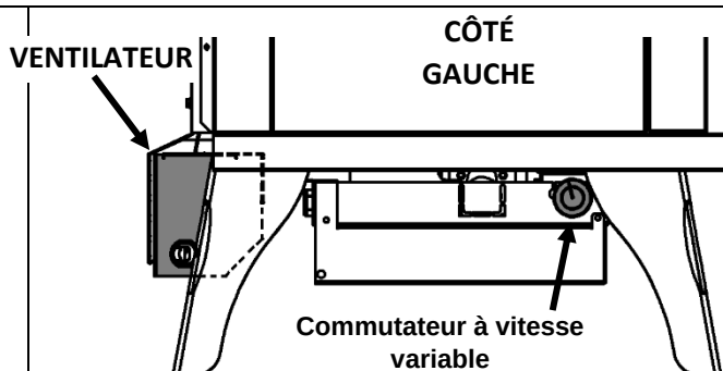
3. Branchez le thermodisque du foyer aux fils du ventilateur avec les connecteurs noirs isolés. Installez le commutateur à vitesse variable et branchez-le avec les connecteurs rouges en plastique.
