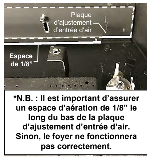
Photo #3 Position inférieure (espace de 1/8")*
