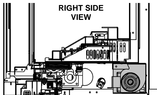
Fan Mount Tabs
