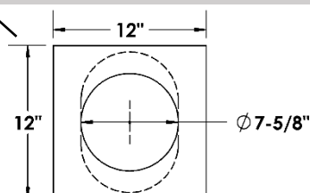
Coupe-feu ZDVFS – Il peut être nécessaire d'allonger le trou selon l'angle du plafond.
