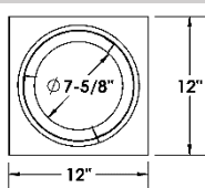
Écran d'isolation pour grenier ZDVAIS ou Z7AIS24
