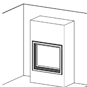
L'enchâssure est construit dans la pièce.
