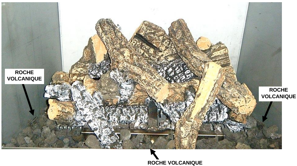
Étape 6 : Placez la roche volcanique sur le plancher de la chambre de combustion et sur le plateau de média. Ne pas placer de roche sur les tubes du brûleur.
