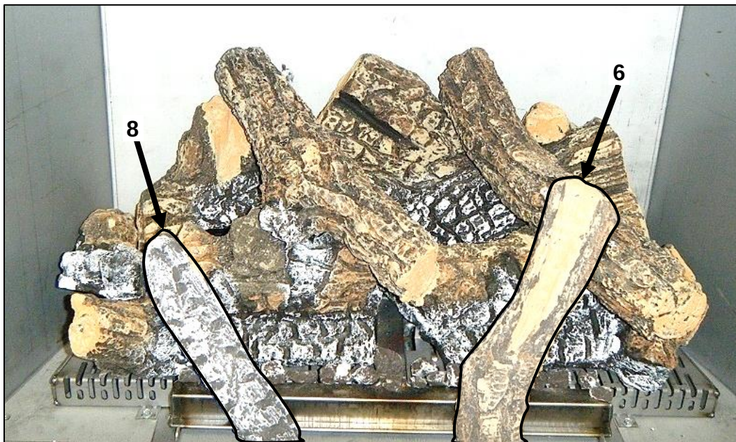
Étape 6 : Placez les bûches 6 et 8 en travers du tube de brûleur avant, tel qu'illustré.
