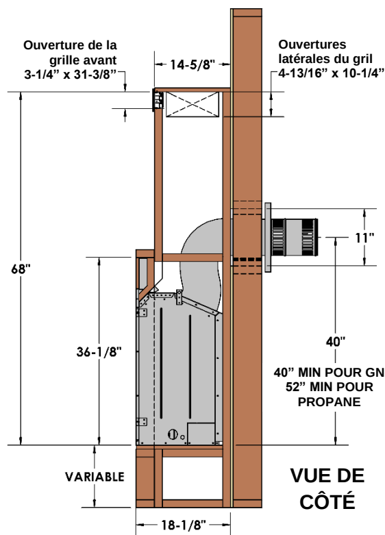
Fig. 1 Charpente l'évacuation horizontale (Voir la section Évacuation à travers un mur)
