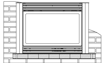
Fig. 2 - Vue avant avec ens. de nivellement
